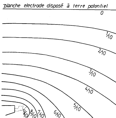
Fig. 2A. La carte d'équipotential. (Lignes sont démembré dixième partie dans espace.)
