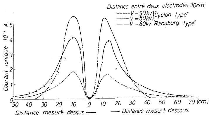
Fig. 8. Diagramme indiquant la distribution de courant ionique.
