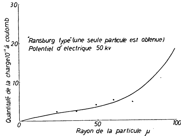
Fig. 14. Relation entre la rayonn de la particule et sa charge.
