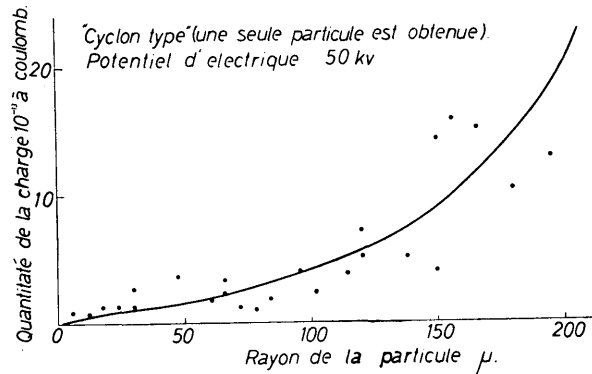
Fig. 13. Relation entre la rayonn de la particule et sa charge.
