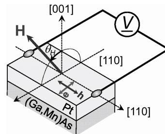
図1. Pt/(Ga,Mn)As 二層膜試料と測定配置の模式図。
