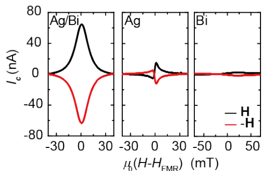
図 3. 強磁性共鳴下におけるスピンプンピング誘起電流量の磁場依存性。
