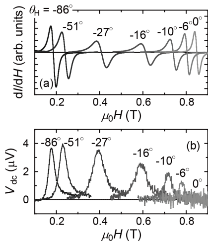
図 2. Pt/(Ga,Mn)As 二層膜における異なる面外磁場角度での FMR スペクトルと電圧信号。
