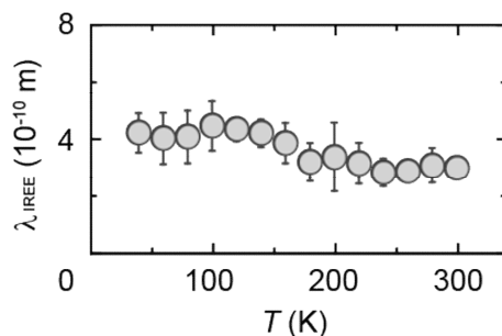
図 4. Bi/Ag 界面におけるスピン流—電流変換効率の温度依存性。
