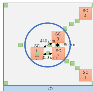
図6 THERMOチップのレイアウトと構成
