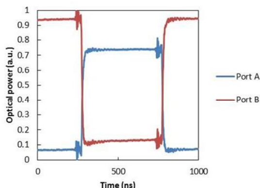
図4：波長選択光スイッチ動特性
