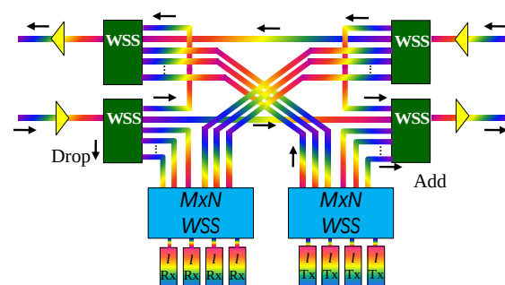
図 11：波長選択スイッチを用いた従来の光ノード構成
