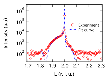
図 8. Pd(100)薄膜の CTR 散乱プロファイル
