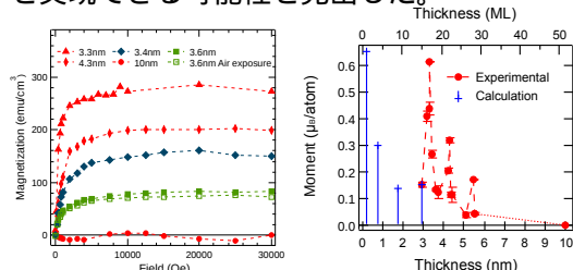
図 6. Pd(100)超薄膜の磁化曲線
