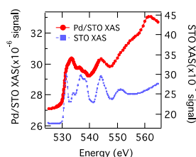
図 4. STO/Pd(100) の XAS
