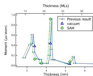
図 10. 表面吸着が生じた際の Pd(100)超薄膜の磁性変化
