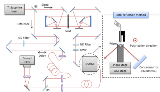
図 1 SI-NSOM 実験セットアップ
