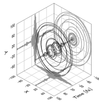
図 8 直交偏光励起における応答関数を用いて励起パルスの偏光整形を行い、円偏光プラズモンを発生させた例
