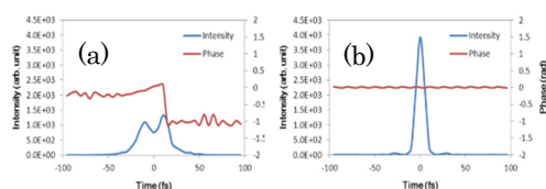
図 10 (a)FTL レーザパルスで励起した際のチップ先端におけるプラズモン波形、(b) 応答関数をもとにチップ先端で FTL が発生するように励起した際のプラズモン波形
