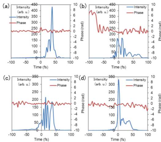
図 5 応答関数に基づき FTL プラズモンパルスが発生するように励起レーザパルスを波形整形した際のプラズモンパルス波形：(a) R=3 , (d) R=2.5 . (c), (d)は(a), (d)の励起パルスでのそれぞれ R=2.5 , 3 におけるプラズモン波形.
