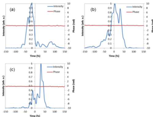
図 6 プラズモン導波路の出力端 1,2,3 においてそれぞれ FTL プラズモンパルスを出力するように励起レーザパルスを波形整形した際の各出口でのプラズモンパルス波形
