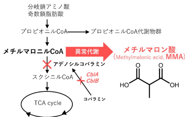
図1 メチルマロン酸産生機構
