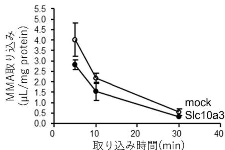
図4 rSlc10a3 発現細胞を用いたメチルマロン酸取り込み実験
