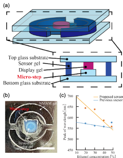
図1 機械的な変位拡大機構を有する構造色ハイドロゲル生化学センサ
