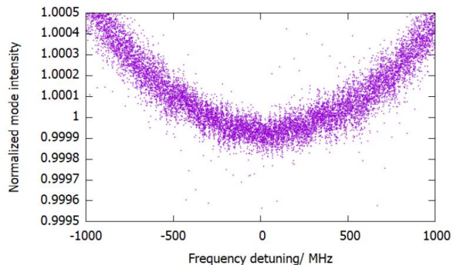
図2: コム直接分光による二重共鳴スペクトル線の観測例。
