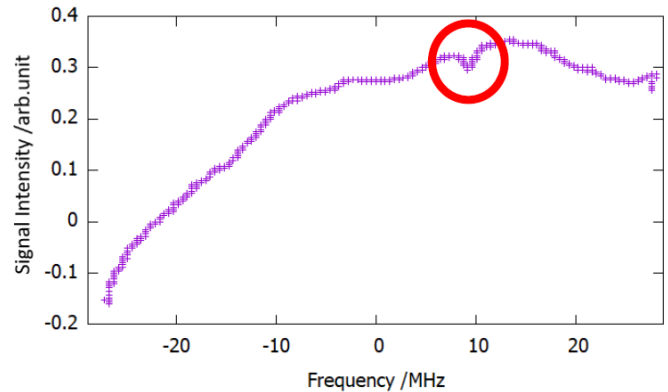
図1: メタン二重共鳴スペクトル線の観測例。赤丸で示した部分が二重共鳴スペクトル線を表す。
