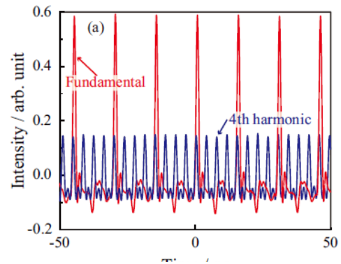
図 5: 4 倍高調波モード同期のパルス(青)と基本モード同期のパルス(赤)。
