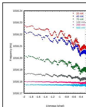
図 6: バイコール多孔質ガラス中固体 ^4\text{He} を入れたねじれ振子の共振周波数の、DC 回転角速度の逆数依存性。0.2 K 以下で周期的に振動する。
