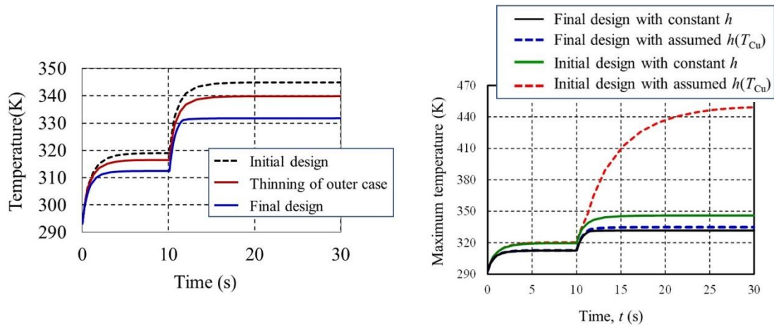
図6 設計改良による最高温度の低減と有効性の検証結果
