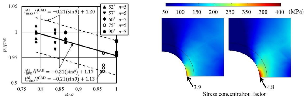
(a) リガメント長さや積層角度の相関性 (b) CAD データ(左)と幾何的精度を考慮した FEA 図 3 アルミ合金製円孔つきダンベル試験片
