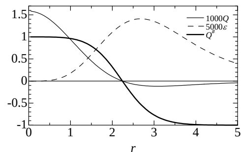
図 5 バーガーズ渦に対する第 2 不変量 Q 、エネルギー散逸率 \epsilon 、コヒーレント構造関数 Q^\# の解析解
