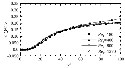
図 4 チャネル乱流におけるコヒーレント構造関数 Q^\# の分散の壁方向分布
