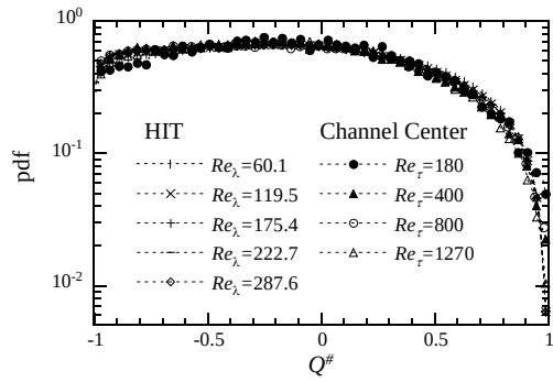
図 2 一様等方性乱流 (HIT) とチャネル乱流におけるコヒーレント構造関数 Q^\# の確率密度関数 (pdf) の分布
