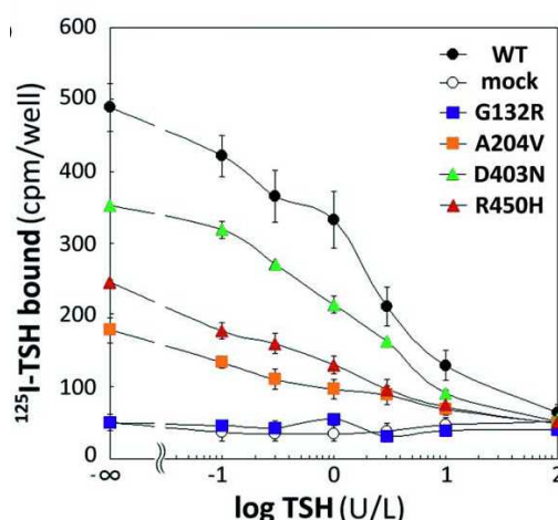
図 変異 TSHR 遺伝子の機能解析: COS-7細胞表面の変異 TSHR への125I-TSH結合能 横軸は細胞に添加したTSHの濃度、縦軸は細胞表面の変異 TSHR へのTSH結合能である。G132R, A204V, D403N, R450Hはいずれも野生型に比してTSH結合能低下を認める(雑誌論文⑥より)。
