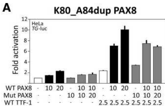
図 変異 PAX8 遺伝子の機能解析：HeLa 細胞を用いた転写活性能
