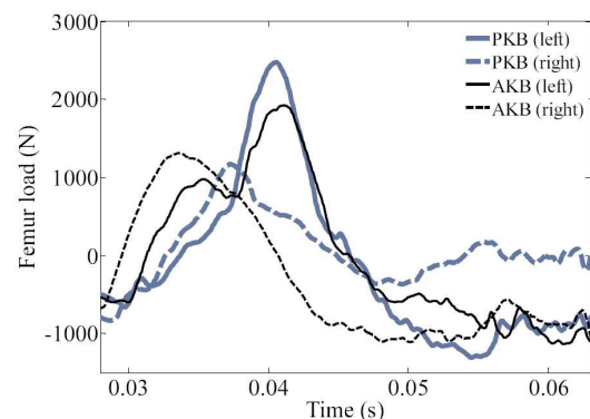
(d) Femur load
