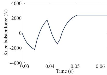
(d) Knee bolster force
