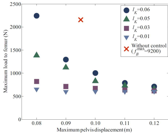
図2 最大ラップベルト荷重 6000 N の場合の腰変位拘束と大腿骨荷重最大値の関係 (×:最大ラップベルト荷重 9200 N、膝部初期クリアランス 0.06 m)
