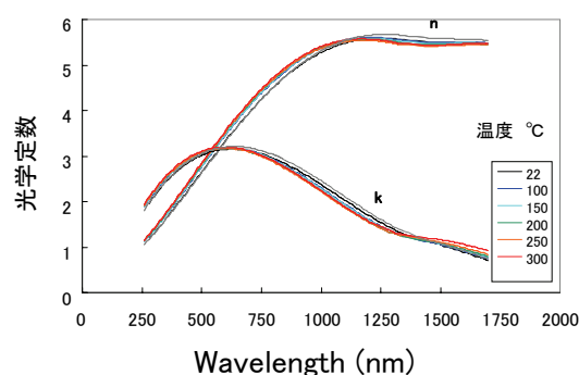
図1：結晶 \text{Ge}_1\text{Sb}_2\text{Te}_4 の複素屈折率
