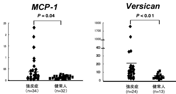
図4. 強皮症、健康人由来単球における MCP-1 と versican の mRNA 発現
