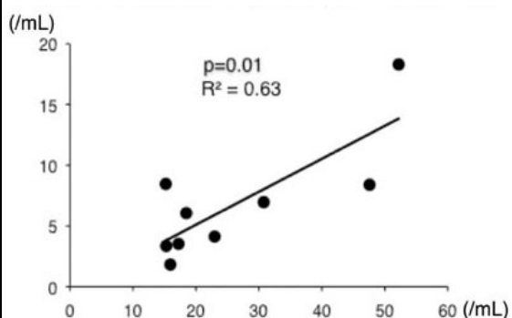
図 1. 7AAD 処理をした MACS 法とロゼット法により得られた CEP 数の相関
