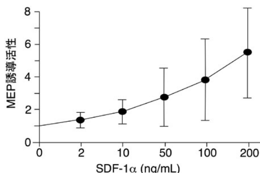
図 2. SDF-1 \alpha 添加により濃度依存性に上昇する MEP 誘導活性
