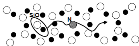
図 1 酸化膜中の SiO 拡散と窒素の影響
