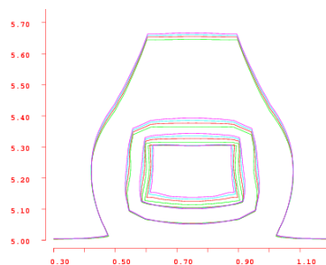
図5 酸窒化シミュレーション結果。2 回目の酸化時間が 0 分（緑）、10 分（赤）、20 分（シア）、30 分（マゼンタ）。1 目盛り 10nm。
