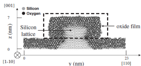
図4 シリコン細線酸化構造
