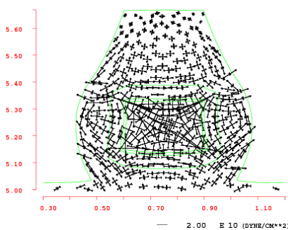
図6 酸窒化シミュレーションから得られた応力分布。
