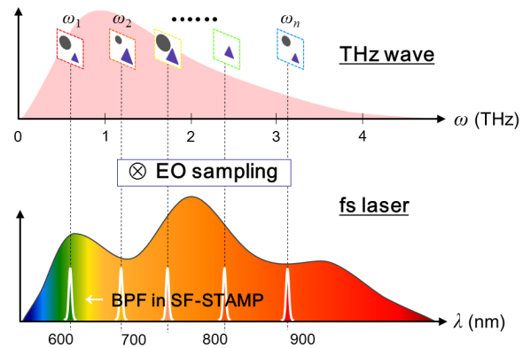
図 2 周波数チャープした THz 波でプローブした周波数毎のイメージを EO 効果を介して周波数チャープした光パルスの周波数成分に転写する概念図
