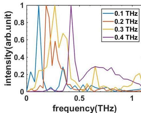
図 6 作成した MHA バンドパスフィルタの透過スペクトル
