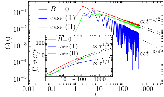
図1: Case 0-IIの時間相関関数
