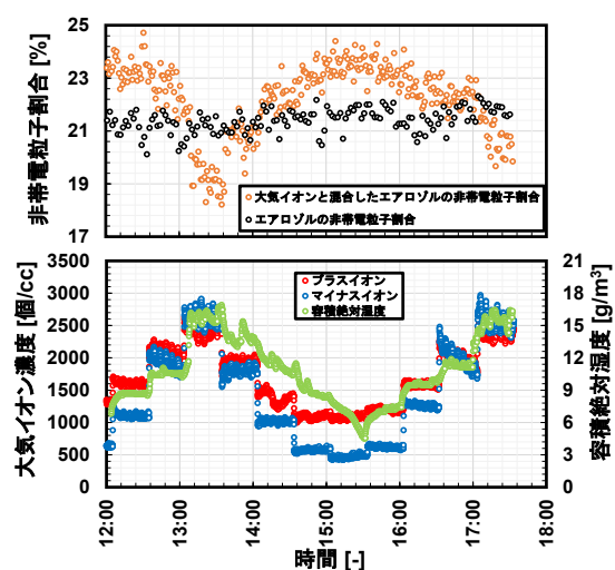
Fig. 5 人為的に容積絶対湿度を変化させた場合の大气イオン濃度と非帯電粒子割合の変動(対象粒径: 0.3\text{--}0.5 \mu\text{m} )
