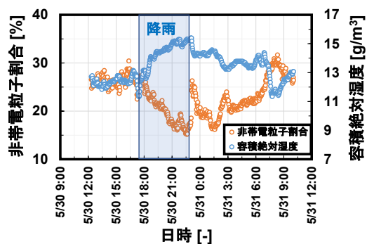
Fig. 3 雨天時の非帯電粒子割合の連続測定 (測定期間: 2018/5/30~2018/5/31, 測定地点: 横浜市, 対象粒径: 0.3\text{--}0.5 \mu\text{m} )
