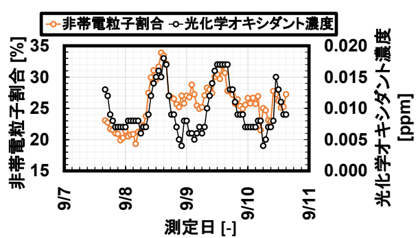
Fig. 4 晴天時の非帯電粒子割合の連続測定 (測定期間: 2018/9/7~2018/9/10, 測定地点: 横浜市, 対象粒径: 0.3\text{--}0.5 \mu\text{m} )
