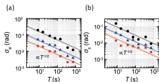
図4：(a) 方位角と(b) 楕円率角の標準偏差の計測時間依存性〔「雑誌論文①」より引用〕。●は、195.3901 THzの周波数成分のデータを表す。▲(■)は、195.3901 THzの周波数近傍の10本(100本)の光コム信号のデータを平均化したデータを表す。
