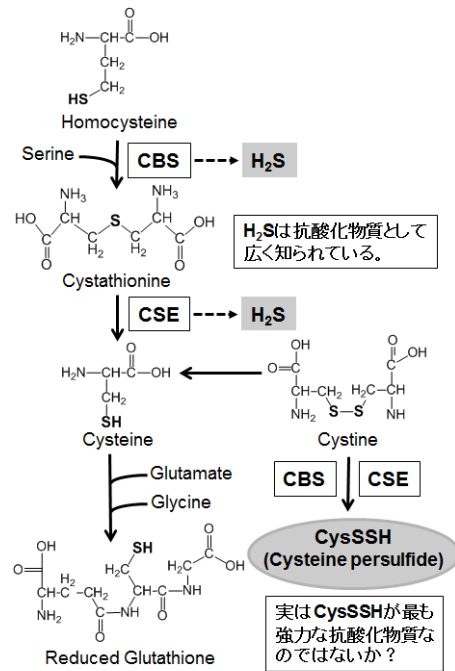
(図1) 含硫アミノ酸代謝経路
