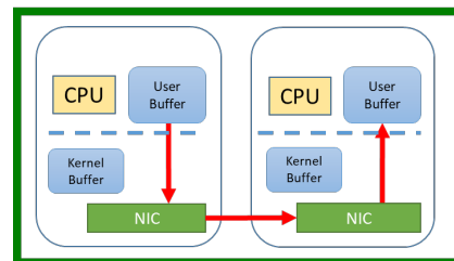
図 2 RAMP + RDMA
