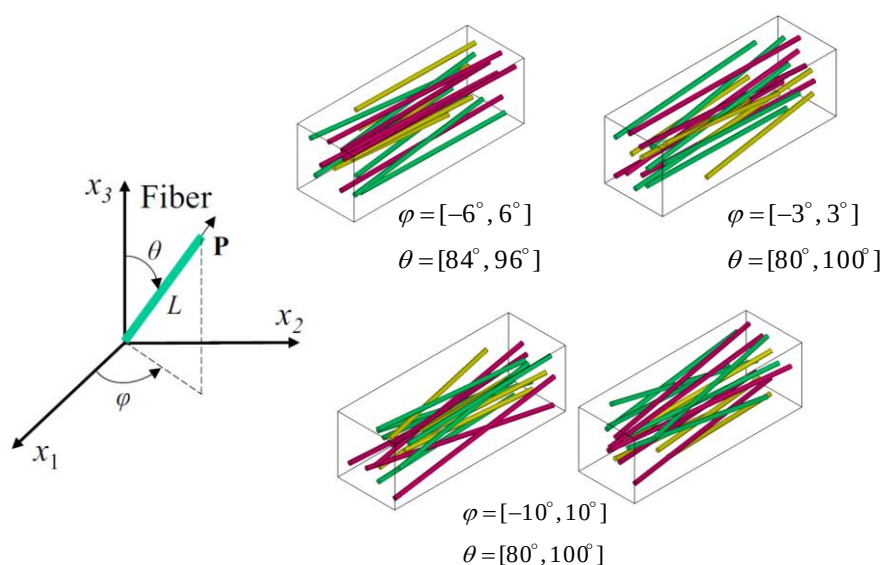
図 1 短繊維強化複合材料のミクロ構造モデル（繊維配向、繊維配置の違いを有するモデル）
