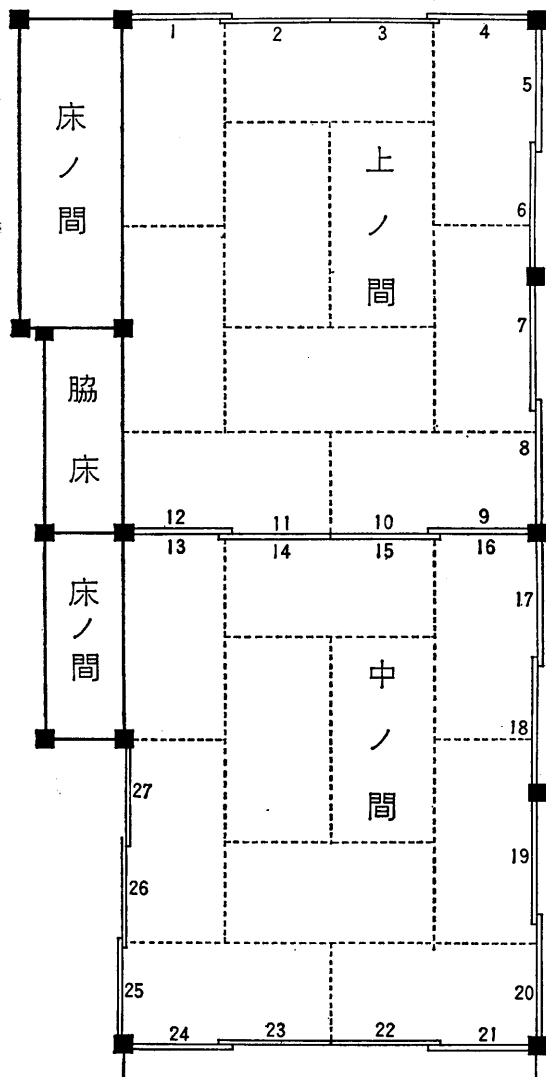
(書院平面図)
