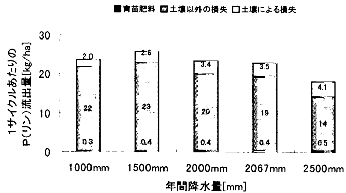
図10 P(リン)の正味流出(投入)量
