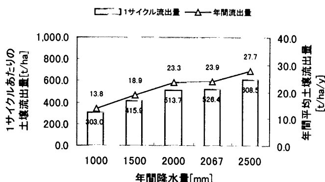
図5 年間降水量に対する土壌流出量の推定
