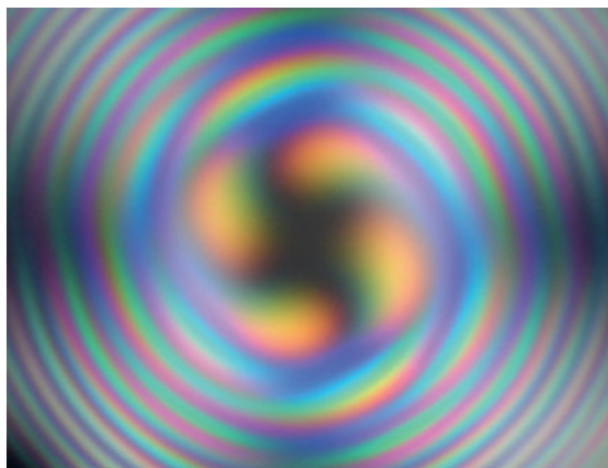
図10. 右水晶板の上に左水晶板を重ねたときのコノスコープ像 (水晶板の厚さは各 4 mm, 偏光板は垂直配置)
