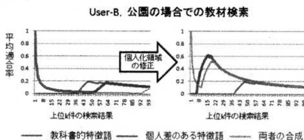
図 8. 知識-体験連結マトリクスの個人化領域の修正による検索精度の向上
