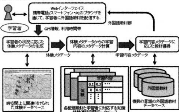
図 3. システムアーキテクチャ：
