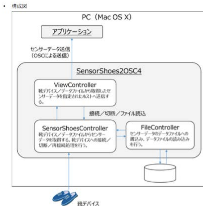
図 4.14: SensorShoes2OSC4 の構成図 1
