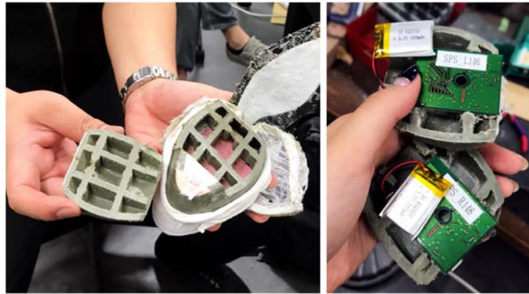
図 4.3: ストーム部分の加工とセンサモジュールの取り付け
