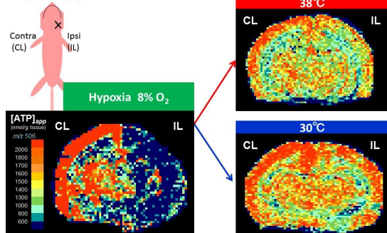
図 1 新生仔低酸素虚血モデル
