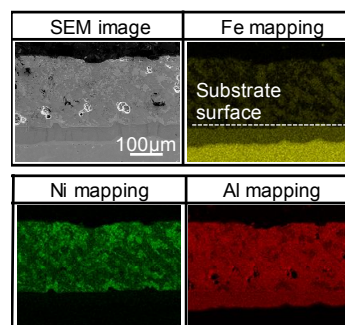
図 2 処理断面の SEM と EDX による分析
