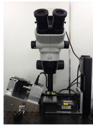
図1. 多層ゲルビーズスポットニング装置
