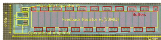
図3 駆動回路を組み込んだ電流電圧変換回路のチップ写真
