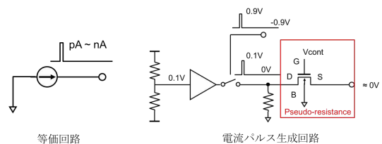
図8 電流パルス生成回路
