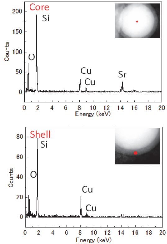
図3 Sr系酸化物コアシェル粒子のEDX結果
