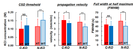
図4 Atp1a2 欠損マウスにおけるCSD感受性と反応性
