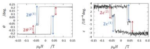
図4 Co(1.2 nm) / Au(3 nm) / Co(0.8 nm) 多層膜の \theta および \varepsilon の磁気ヒステリシス曲線
