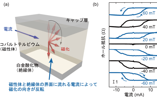
図3. Pt 酸化物によるスピントルク磁化反転。
