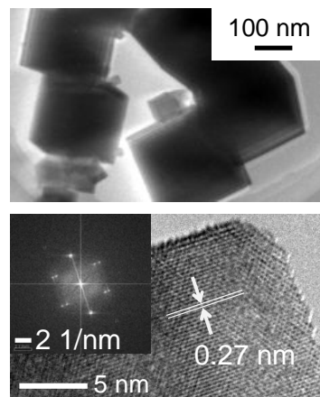
図2 \text{CeO}_2:\text{Sm}^{3+} 試料の TEM 写真
