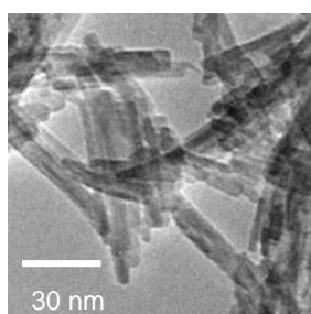
図1 \text{CePO}_4:\text{Tb}^{3+} 試料の TEM 写真
