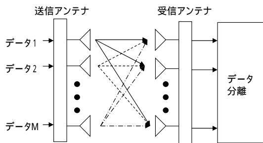
図 1 従来型 MIMO 伝送の概念図
