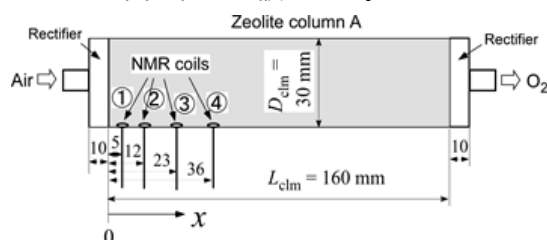
図 1 小型 NMR コイルを挿入したゼオライト吸着筒
