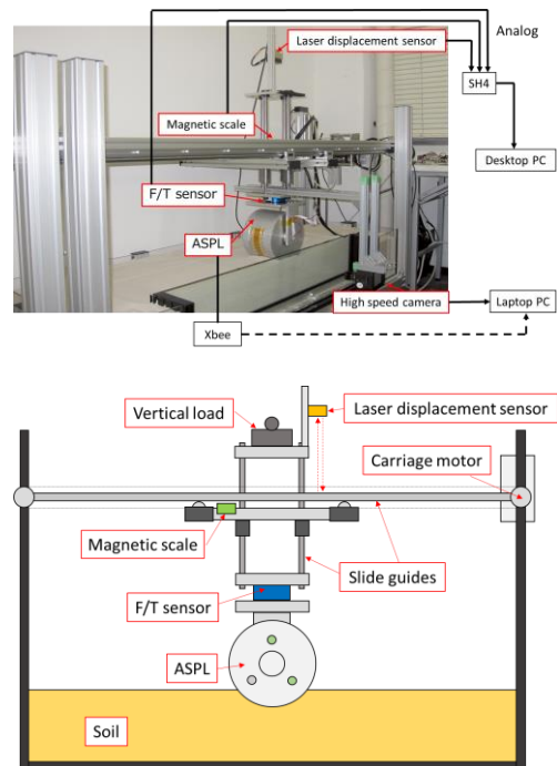
図1：車輪走行試験装置
