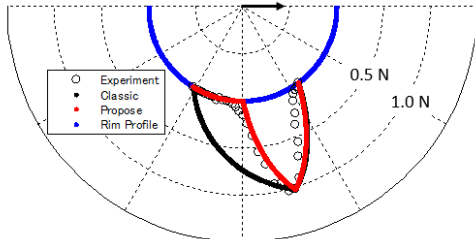
図 6: 車輪圧力分布の修正モデル (丸プロット: 実験結果, 黒線: 従来モデル, 赤線: 提案モデル,)
