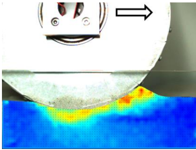
図 5: PIV による砂の流れ場計測 (赤色: 砂の移動が顕著, 青色: 砂が静止状態)
