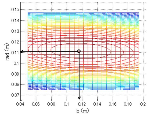
図 7: 車輪最適設計結果 (最適な車輪半径, 幅が等高線プロット上に示される)
