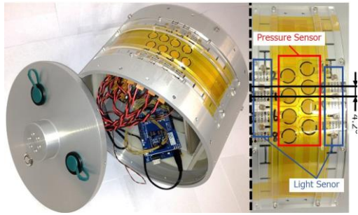
図 2：車輪実装型センサシステム
