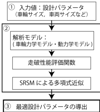
図 3：最適設計フローチャート
