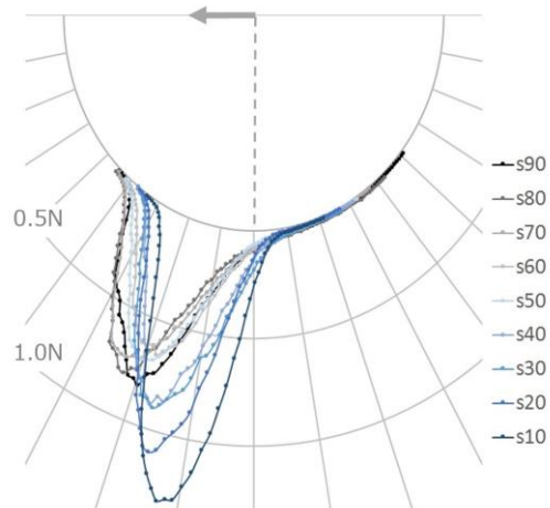
図 4：車輪実装型センサシステム 圧力分布計測実験結果 (車輪の滑りの違いにより分布範囲が異なる)
