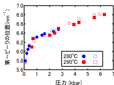
図6 高分子P4MP1 熔融体のX線回折におけるピーク位置の圧力依存性。塗りつぶしたマークは加圧時、白抜きのマークは減圧時のデータを示す[8]。
