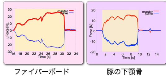
Fig.5 力応答
