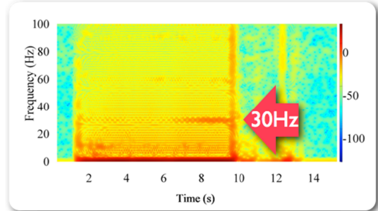
Fig.6 マスタ側 力応答の時間-周波数解析
