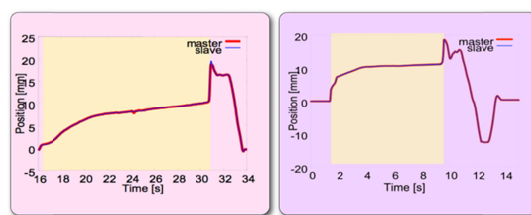
Fig.4 位置応答
