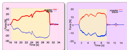
Fig.5 力応答
