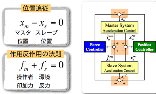
Fig.2 システム構成
