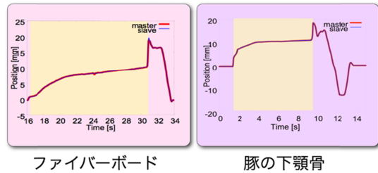
Fig.4 位置応答
