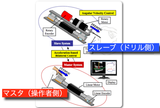
Fig.2 システム構成
