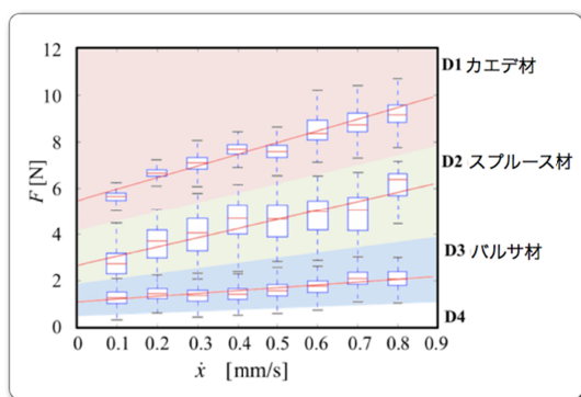
Fig.7 等速度実験結果
