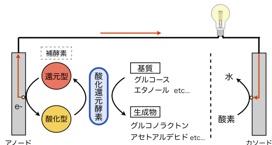
図1 酵素バイオ電池の原理
