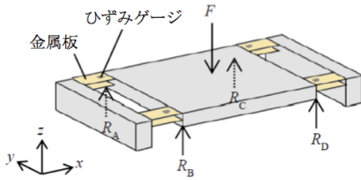
図4 押下位置・力検出装置
