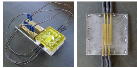
図2 原理確認装置
