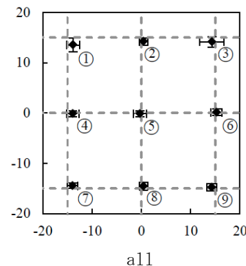
図6 押下位置の実験結果
