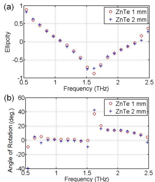
図5: 回転電気光学結晶法で計測した、1/4 波長板を透過させたテラヘルツ波の楕円率(a)と旋光角(b) (学会発表[4]の予稿の図を一部改変)。
