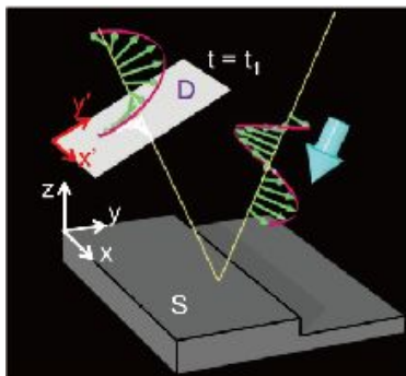
図2：反射型テラヘルツ波イメージング装置による凹凸計測の概念図[5]。
