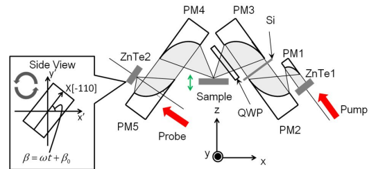
図 1 : 反射型テラヘルツ波偏光顕微鏡の実験装置模式図(産業財産権[1])。
