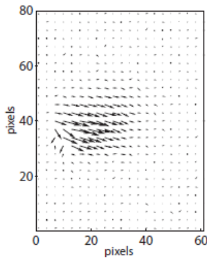
図4: CCD カメラを用いたテラヘルツ電場ベクトルイメージング(学会発表[10]の予稿より)。
