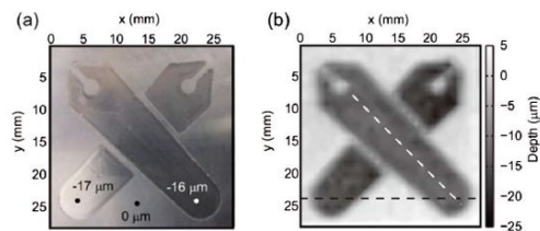
図3：アルミニウム切削加工部品の凹凸計測結果[5]。
