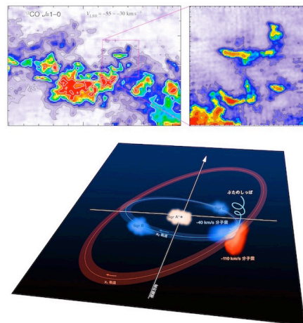
図 3) (a) Sgr C 領域の CO J=1-0 輝線強度図。(b) 「ぶたのしっぽ」分子雲拡大図。(c) 同分子雲の形成メカニズム。
