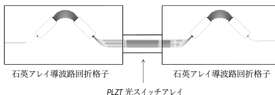
図1：波長選択光スイッチの構成
