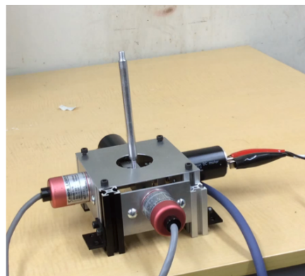
図2 ジョイスティック
