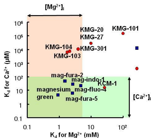
図1 従来のMgプローブとKMGとの比較 Mg選択性でKMGは勝っている
