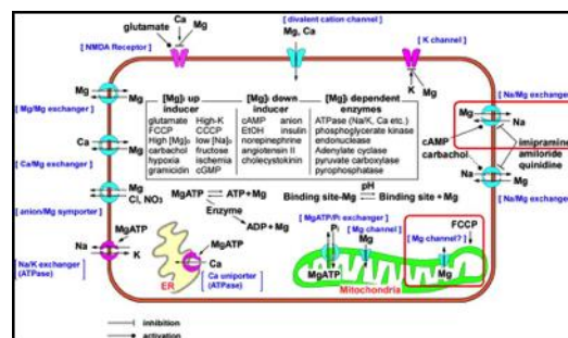
図2 細胞内Mg 2+ 濃度変化を起こすと考えられる種々の要因(過去の文献情報からまとめた)
