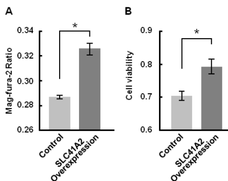
図8 Mg 2+ 輸送体SLC41A2を過剰に発現させた細胞でのMPP + 添加に伴う[Mg 2+ ] i 変化 A: [Mg 2+ ] i 濃度変化、B: 細胞生存率
